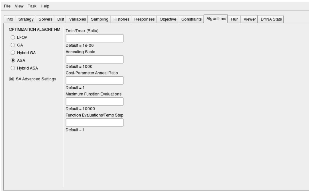
Figure 20-8: Selection of the SA parameters
